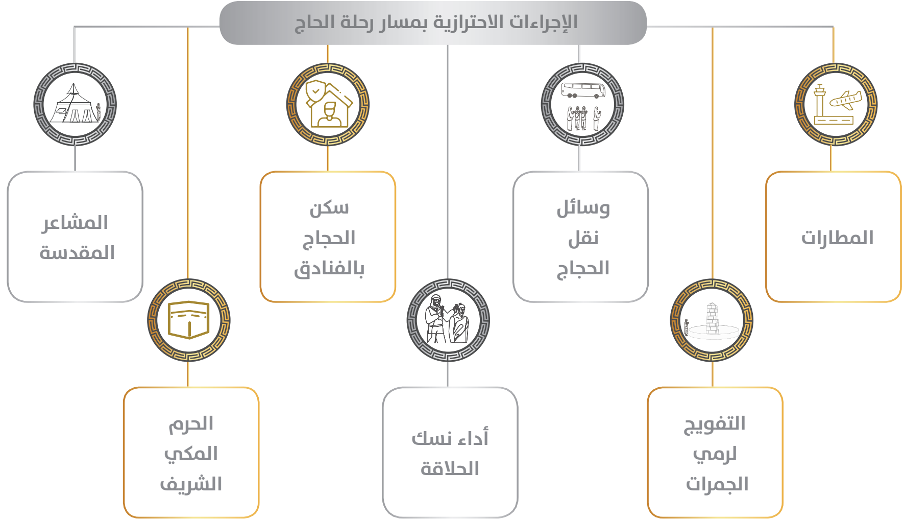
شكل(46): الإجراءات الاحترازية بمسار رحلة الحاج بموسم حج 1441هـ.
